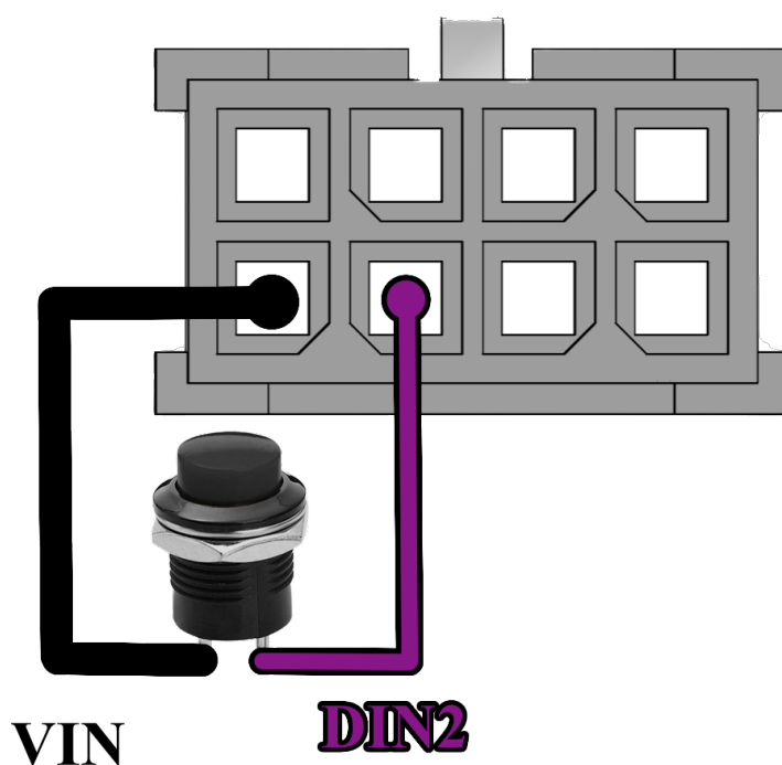
Figura 8: Ligação entrada digital J-R11.
