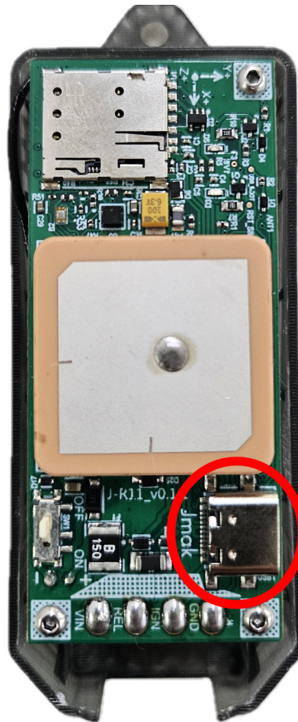
Figura 17: Conexão USB-C do J-R11.
