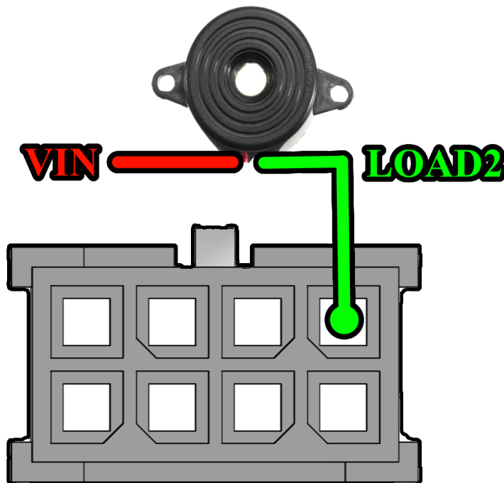
Figura 10: Ligação saída digital J-R11.
