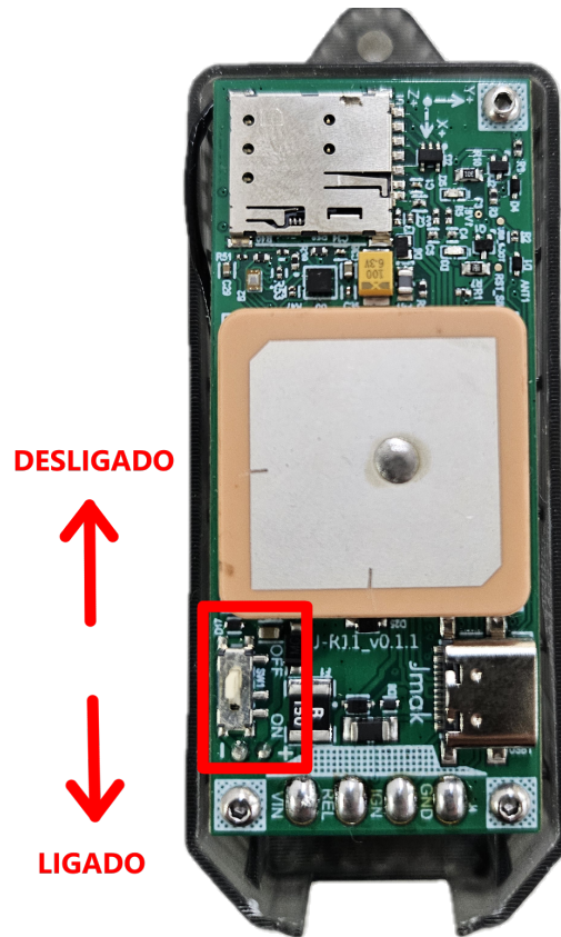
Figura 5: Ligação bateria J-R11
